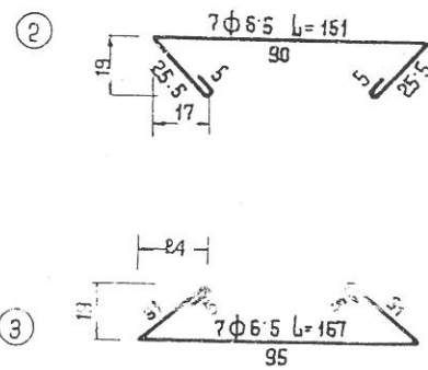
ДЕТАИЛ НА ВРЪЗКА
