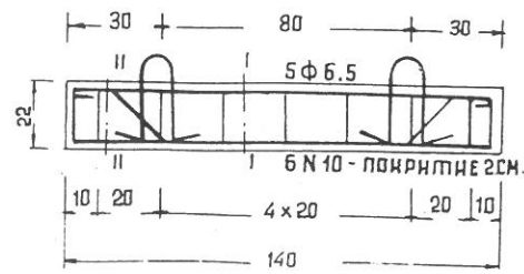
НАДЛЪЖЕН РЪЗРЕЗ
