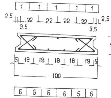
СЕЧЕНИЕ 1-1
