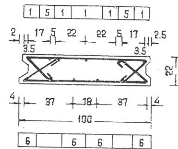
СЕЧЕНИЕ II-II
