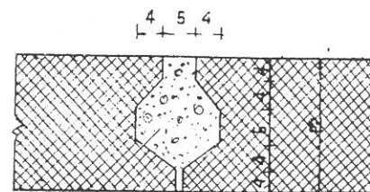
ДЕТАИЛ НА ВРЪЗКА
