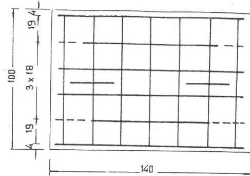
ДОЛНА АРМИРОВКА
